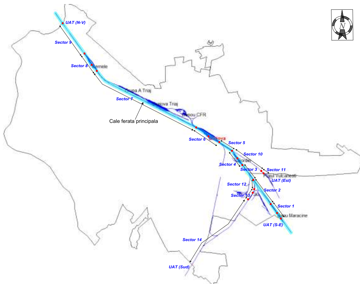
Figura nr 2 Delimitarea segmentelor de cale ferată considerate în cadrul Unității Administrative Teritoriale, cu evidențierea segmentelor de cale ferată principală
