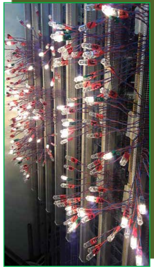
Rama repartitor testare funcționare semnale
